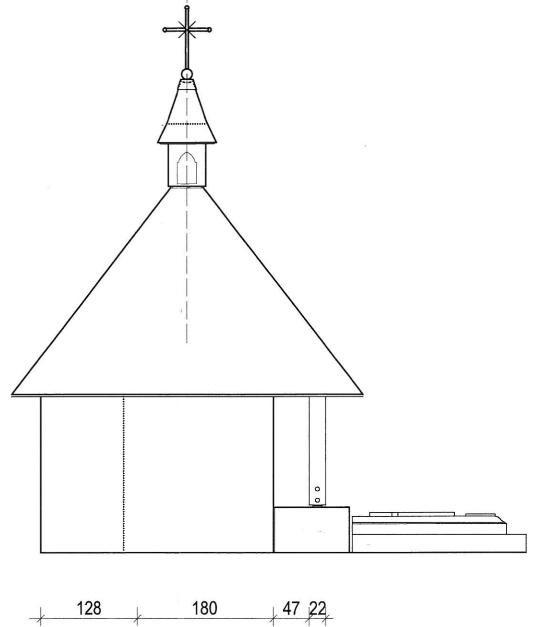
ELEWACJA BOCZNA
