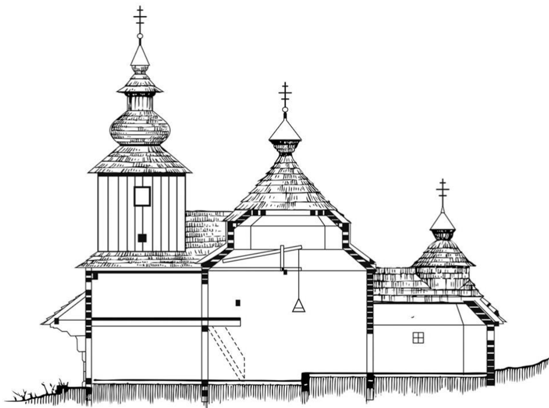
Ryc. 1. Cerkiew pw. św. Michała Archanioła z 1764 r. z Novej Sedlicy – przekrój podłużny (rys. L. Kostulski).
